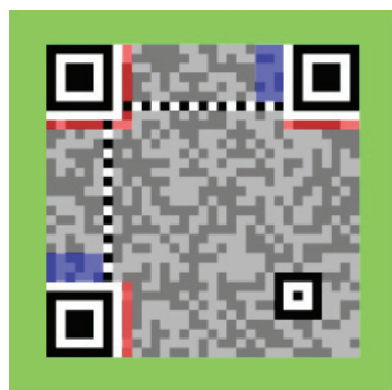
Структура QR-кодов
