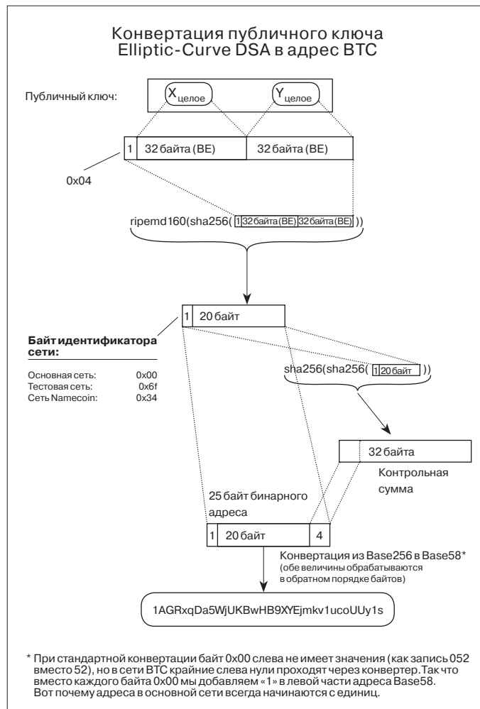
Алгоритм преобразования публичного ключа ECDSA в адрес Bitcoin
