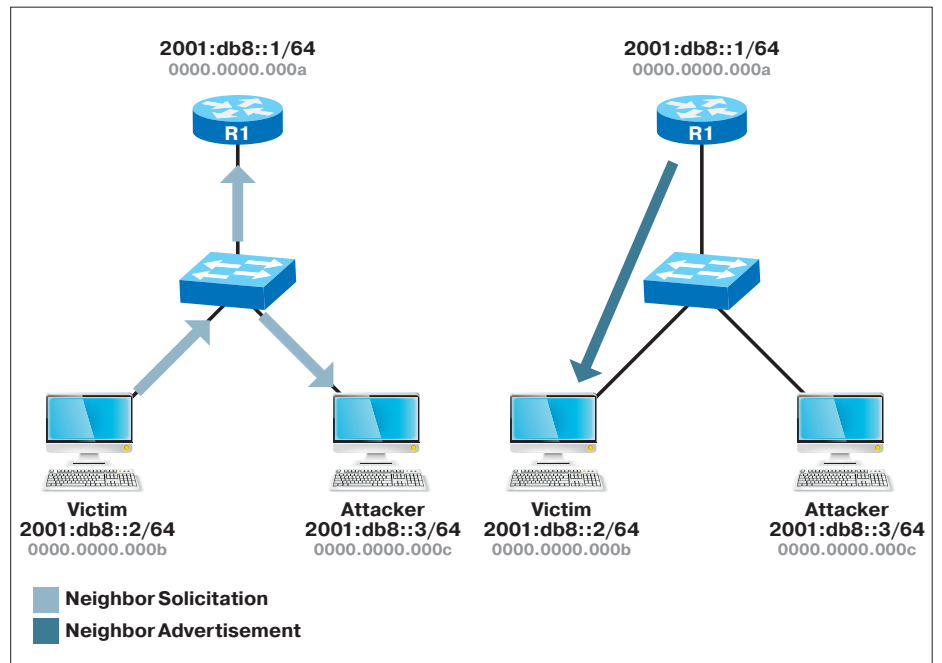
Рис. 1. Протокол NDP
