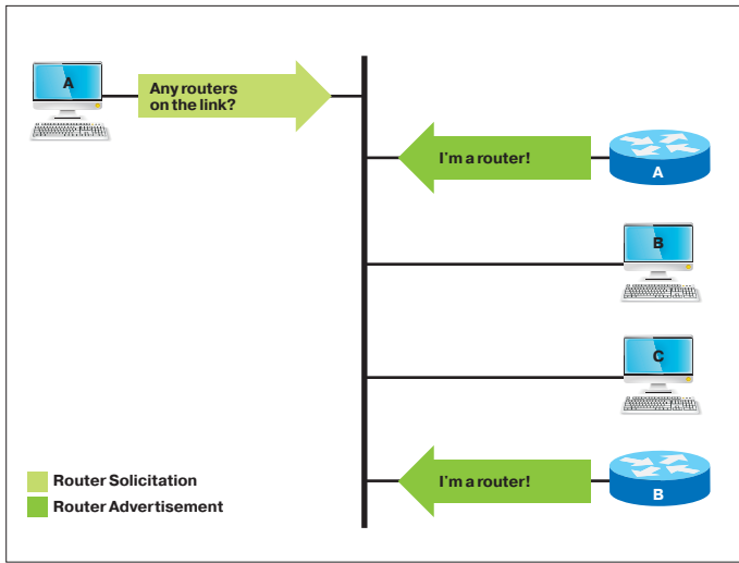
Рис. 3. Легальное применение ICMPv6 Router Advertisement
